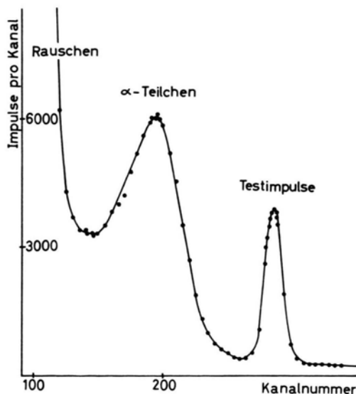
Abb. 1. Impulshöhenspektrum der Po-210 Quelle am InSb-Detektor.
